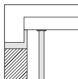
Nahezu boden- gleicher Einbau
