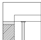
Erhöhter Einbau mit Fliesensockel
